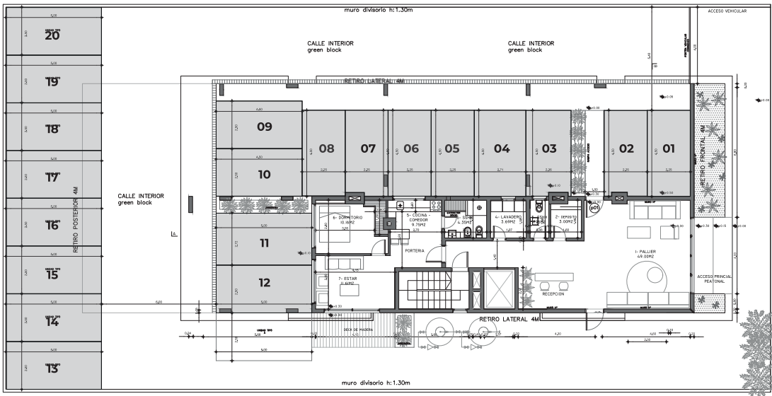
PLANO DE COCHERAS (PLANTA BAJA)
